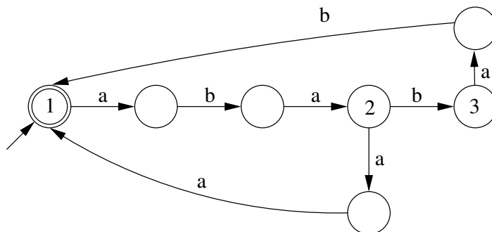
On obtient alors un automate élémentaire équivalent à \mathcal{A} représenté à la figure II.6, les états supplémentaires ne portant pas de numéro.
