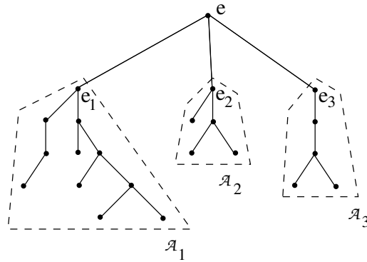
FIGURE VI.1. Un arbre.
